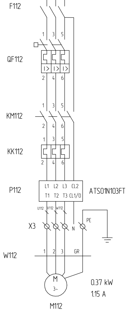
рольганг 112
