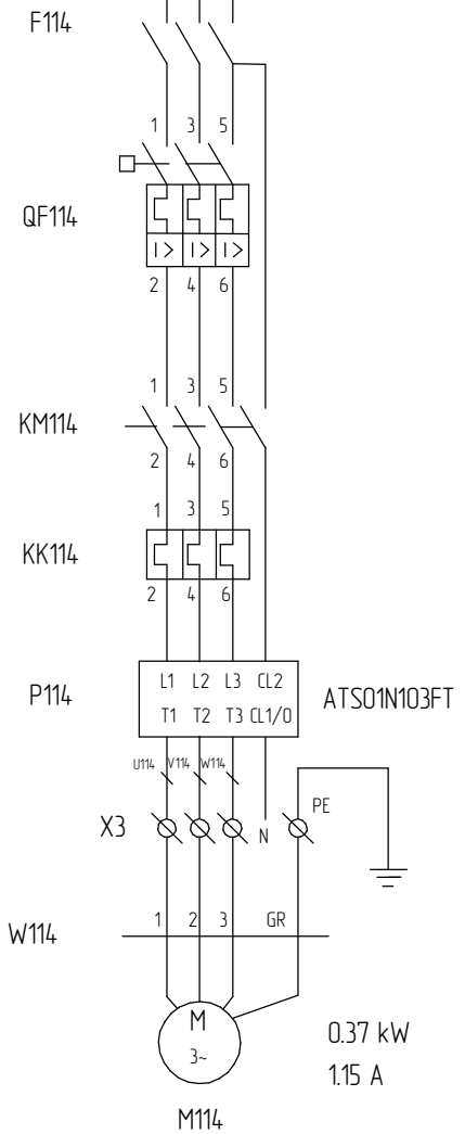
рольганг 114
