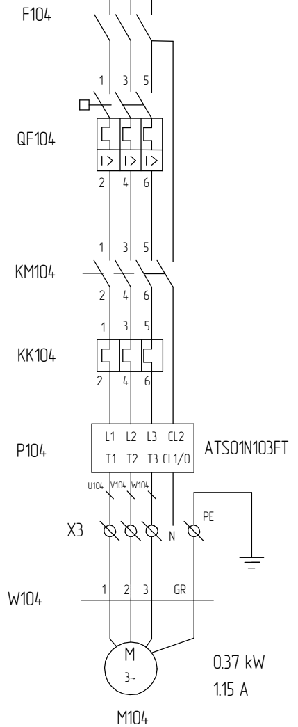
загрузка паллет рольганг 104
