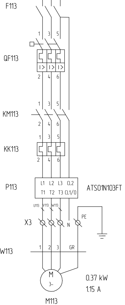
рольганг 113
